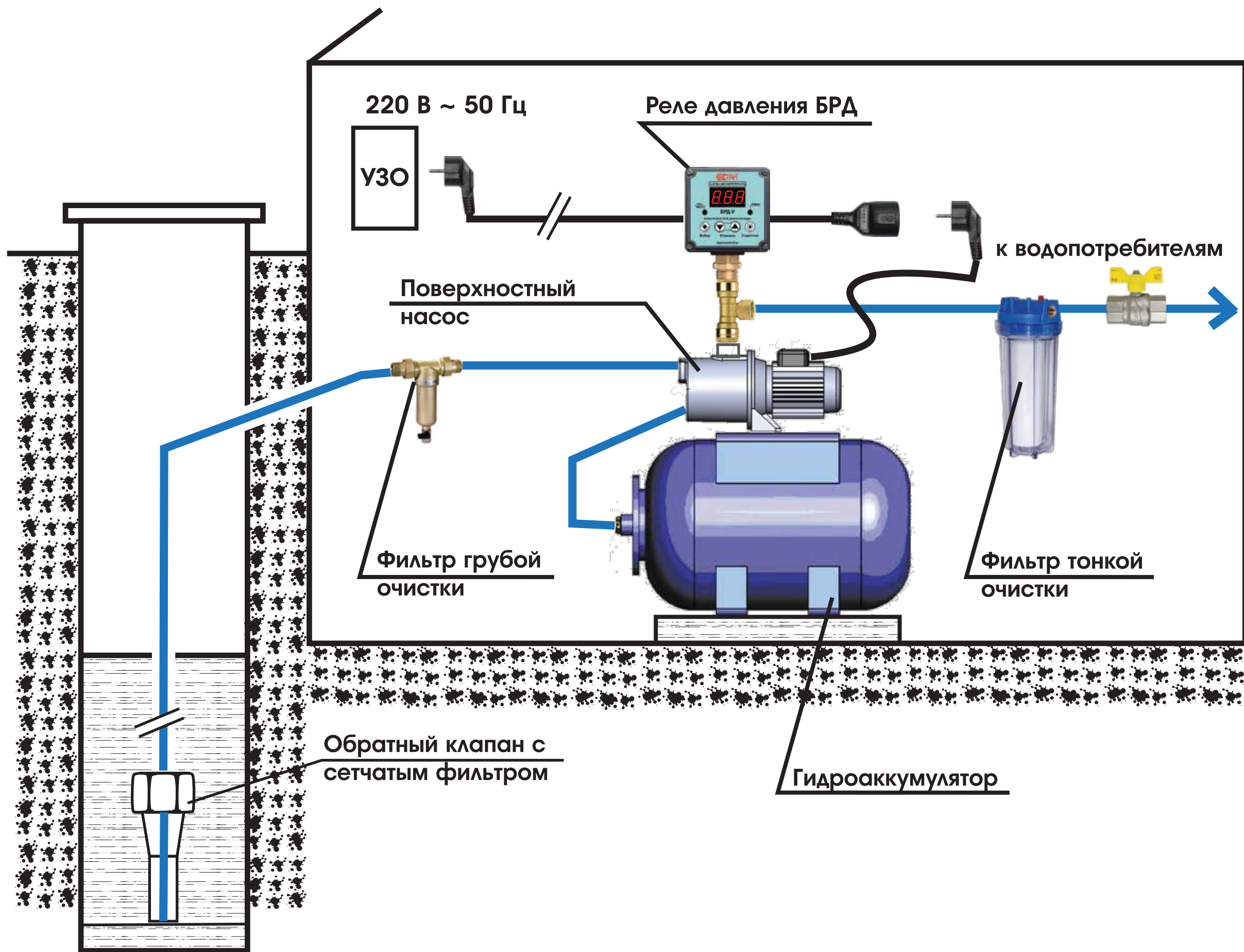
Схема 1. Подключение реле давления БРД-У “Акваконтроль” с поверхностным насосом
